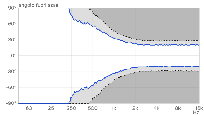
Linee di uguale pressione sonora. Blu: -6 dB. Tratteggiata: -12 dB. La regione bianca si mantiene entro 6 dB dall'asse.
