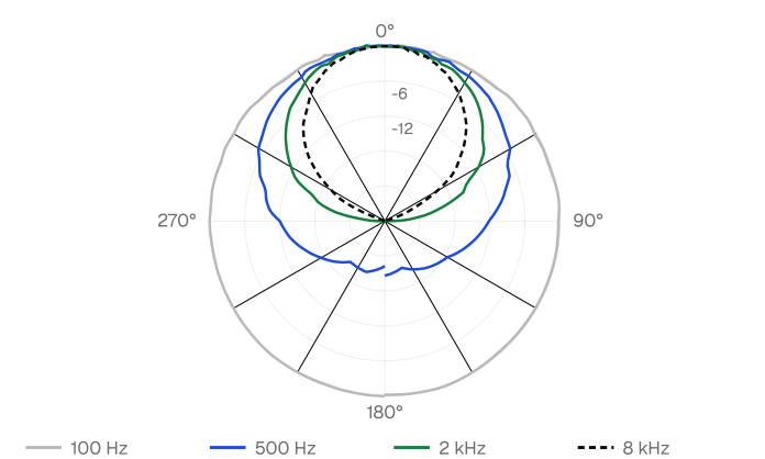
Normalizzata sull'asse. Anelli a intervalli di 6 dB fino a un centro di -30 dB. Potenza in banda 1/3 di ottava.
