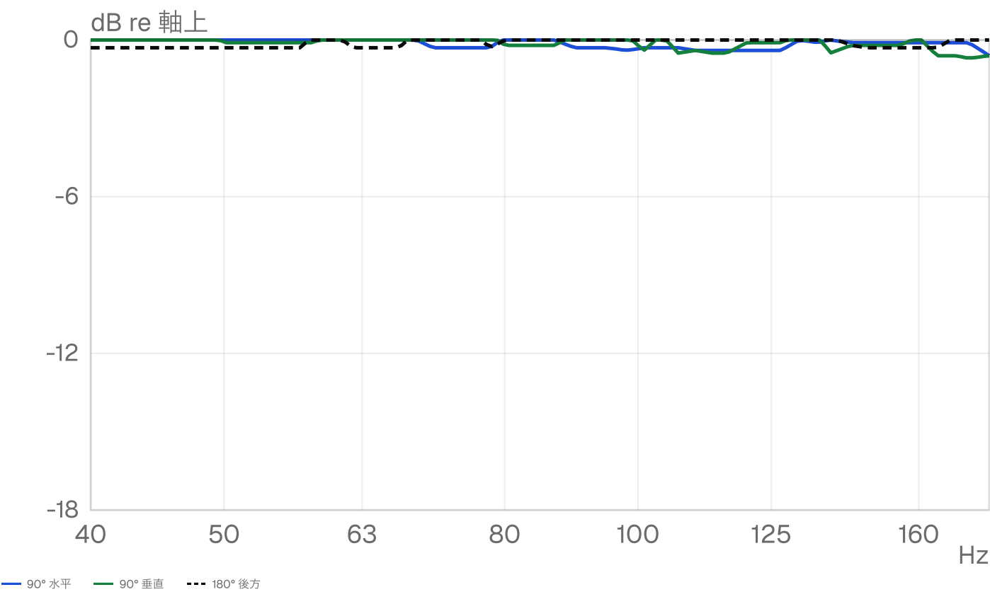
周波数に対する軸外減衰
