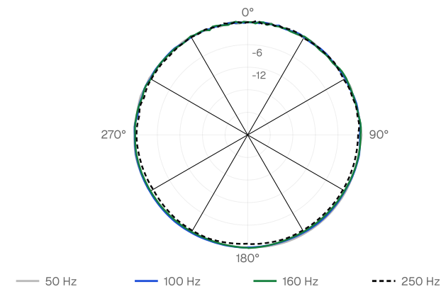
ポーラー応答、垂直
