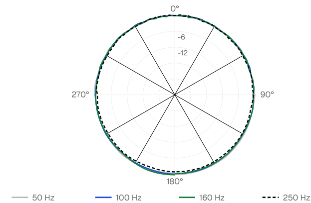
ポーラー応答、水平
