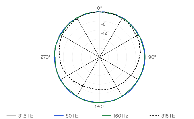
ポーラー応答、垂直
