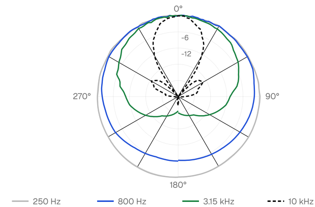
폴라 응답, 수평
