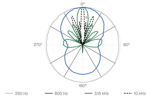
폴라 응답, 수직
